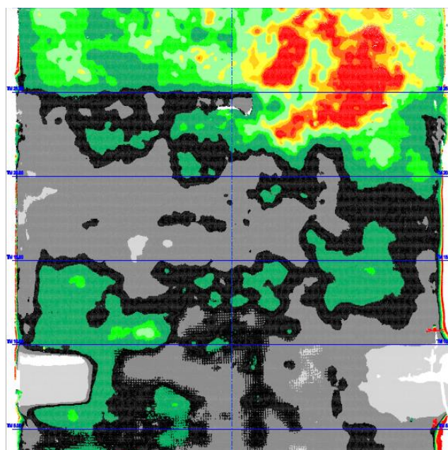
Flächenhafte Profilkontrolle Verzweigungskaverne Vispertaltunnel, VS.
